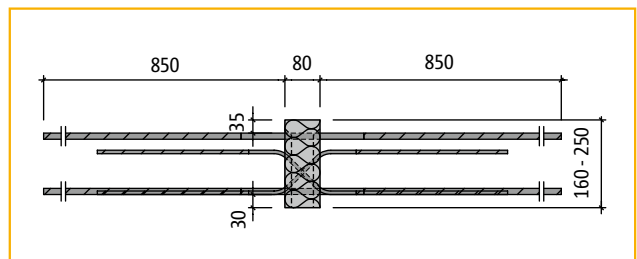
Schöck Isokorb® type D70-CV35
