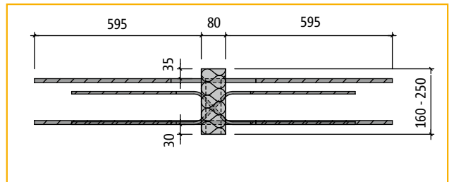
Schöck Isokorb® type D30-CV35
