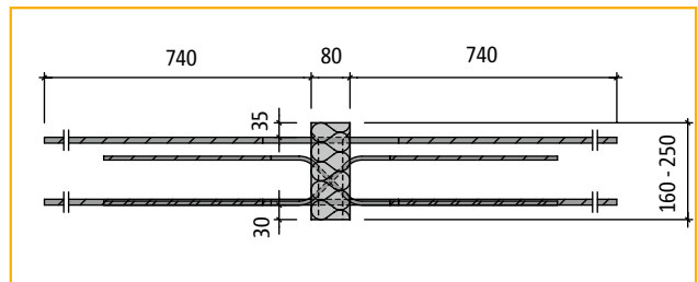
Schöck Isokorb® type D50-CV35
