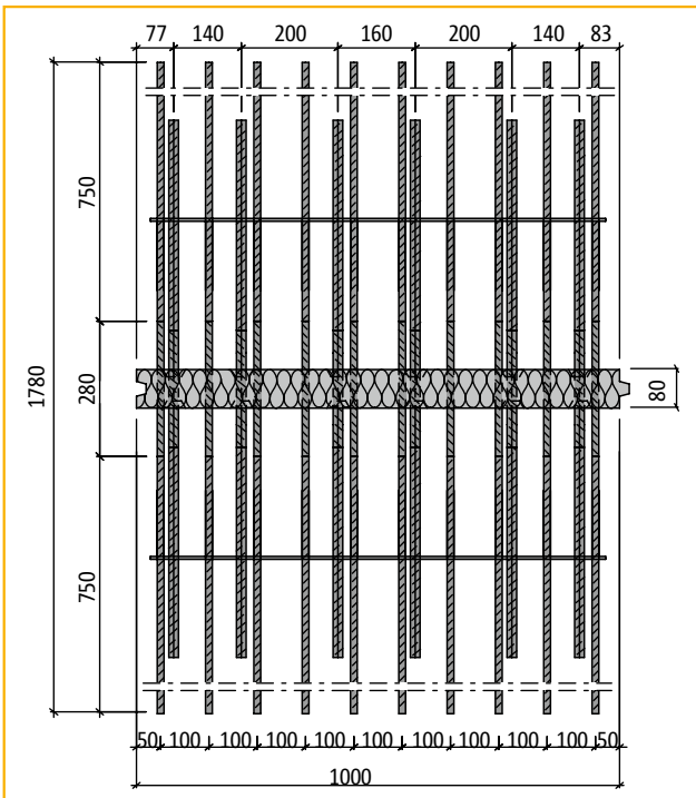
Bovenaanzicht Schöck Isokorb® type D70-CV35
